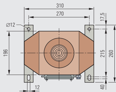
Plano de dimensiones 22
