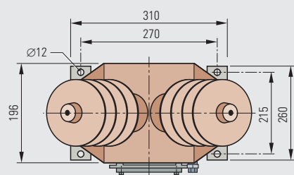
Plano de dimensiones 24
