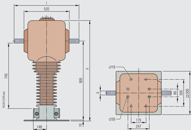
Plano de dimensiones 15
