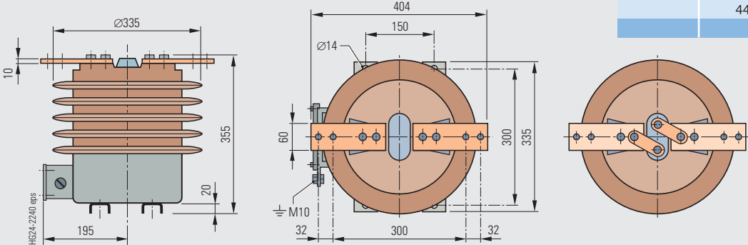
Plano de dimensiones 10
