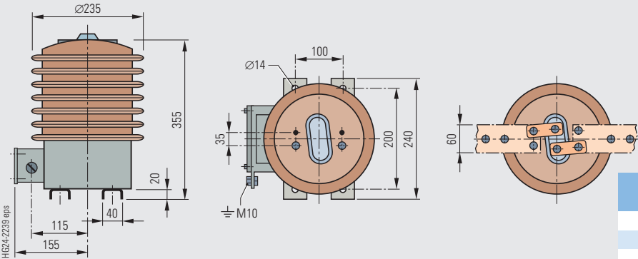
Plano de dimensiones 9
