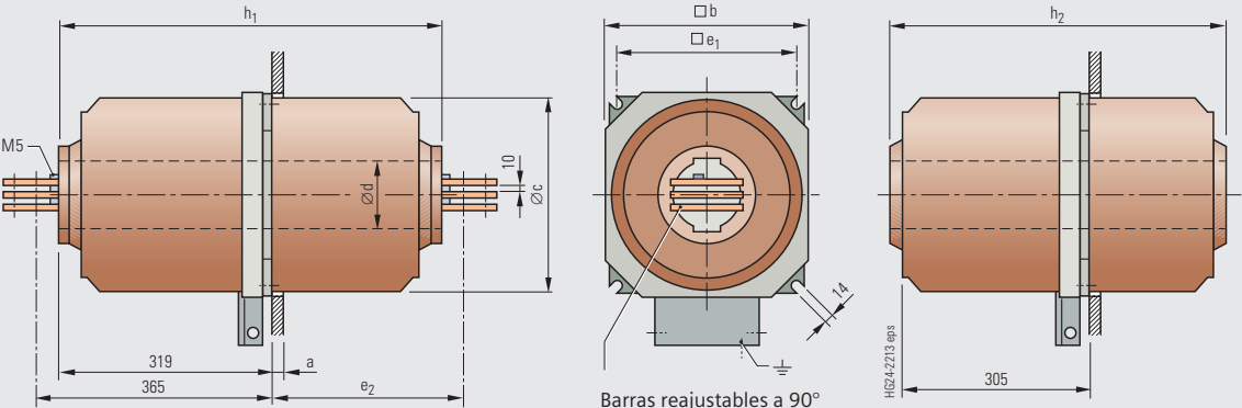
Plano de dimensiones 8
