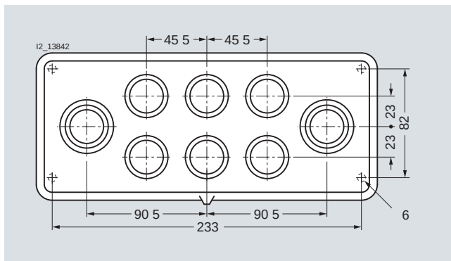
8HP1 512-1
