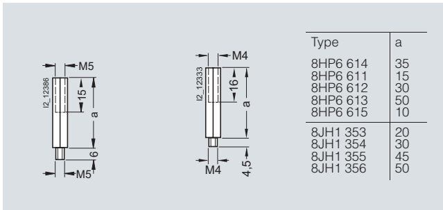
8HP6 6.. M5 stud bolt
