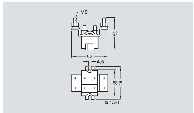
8JH4 044
