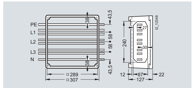
2 x Cu (30 x 10) mm, 1000 A
