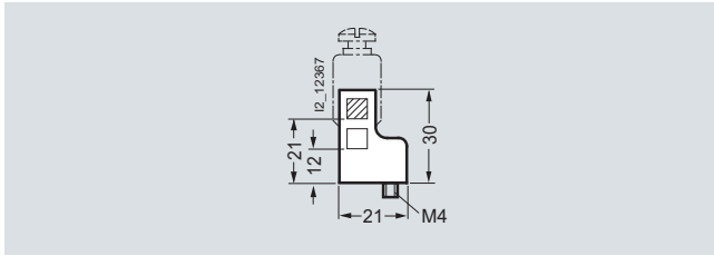
8JH4 230
