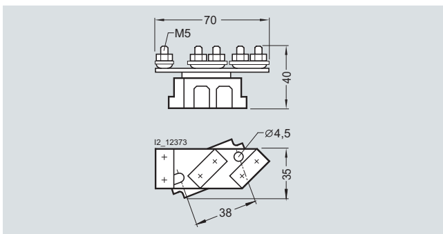
8JH4 043
