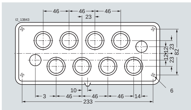
8HP1 513-1
