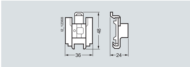
8HP6 601
