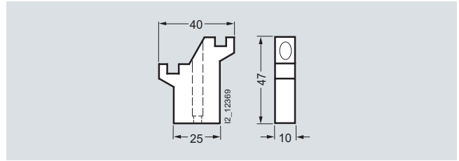
8GF9 320-1
