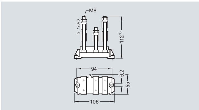
8JK4 06, 8JK4 061 1)
