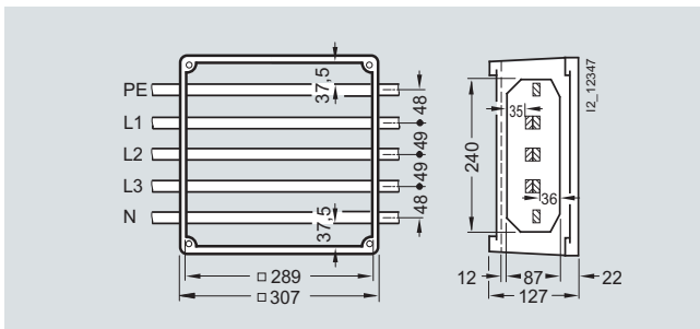
Cu 20 x 8 mm and 2 x Cu (20 x 8) mm, 400 A and 630 A
