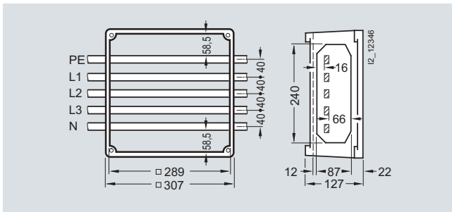
Cu 12 x 5 mm, 250 A and CU 2 x 12 x 5 mm, 400 A
