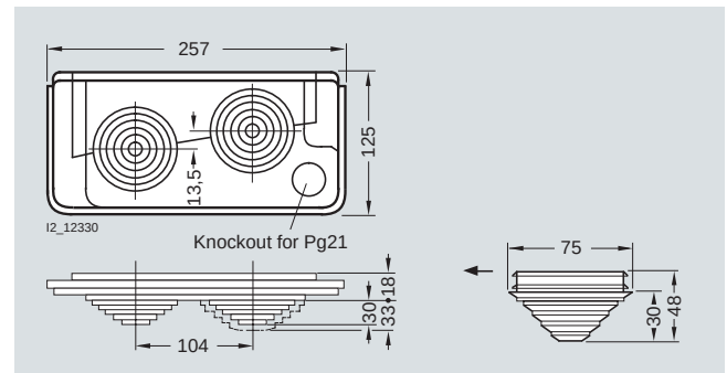
8HP1 520
