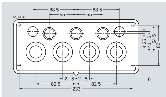
8HP1 511-1
