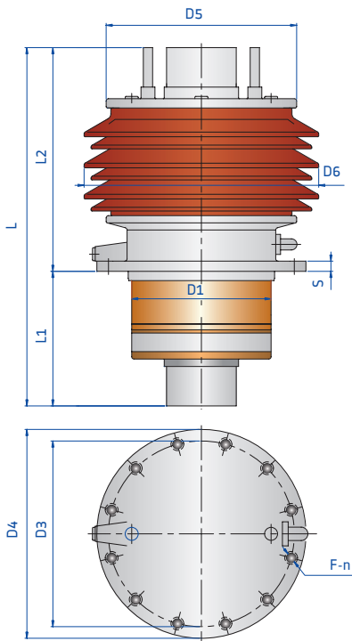
Fig. 3: PTFR dimensions
