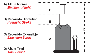
Gatos Hidroneumáticos Hydroneumatic Jacks
