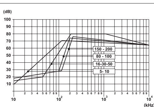
Attenuazione di modo differenziale Differential mode attenuation
