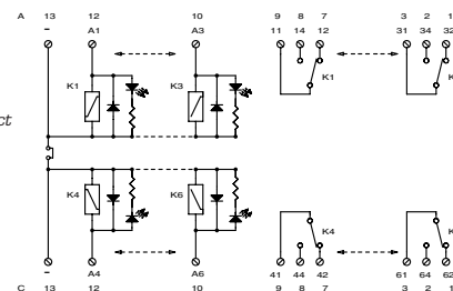
1 Contatto Scambio 1 Changeover Contact EMR6X1...
