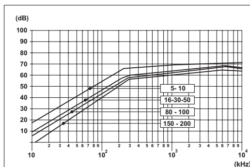
Attenuazione di modo comune Common mode attenuation
