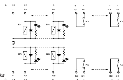
1 Contatto NA 1 NO Contact EMR8X1...
