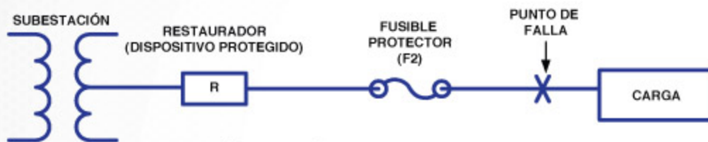
Figura 8. Coordinación Restaurador Fusible
