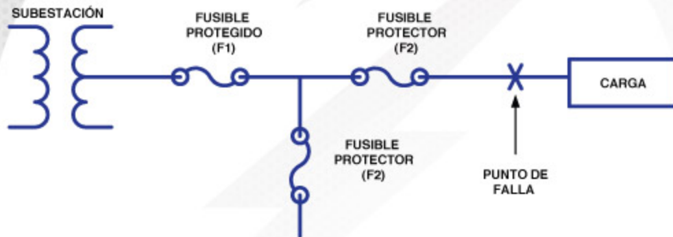
Figura 7. Coordinación Fusible - Fusible
