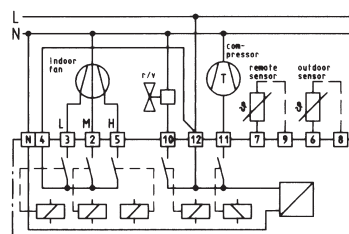
Instat 7 52755 – für Wärmepumpe m. Umkehrventil Instat 7 52755 – for heat pumps with reverse valve
