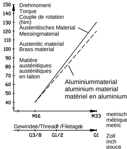
Einschraubgewinde Screw-in thread Filetage à visser
