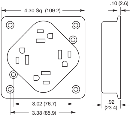
Quadplex® Receptacle
