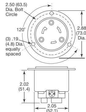
70530MB and 70530ER
