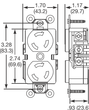
4700DR, 70615DR and 4750DR
